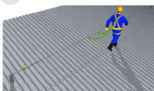
LINHA DE VIDA EM TELHADO
